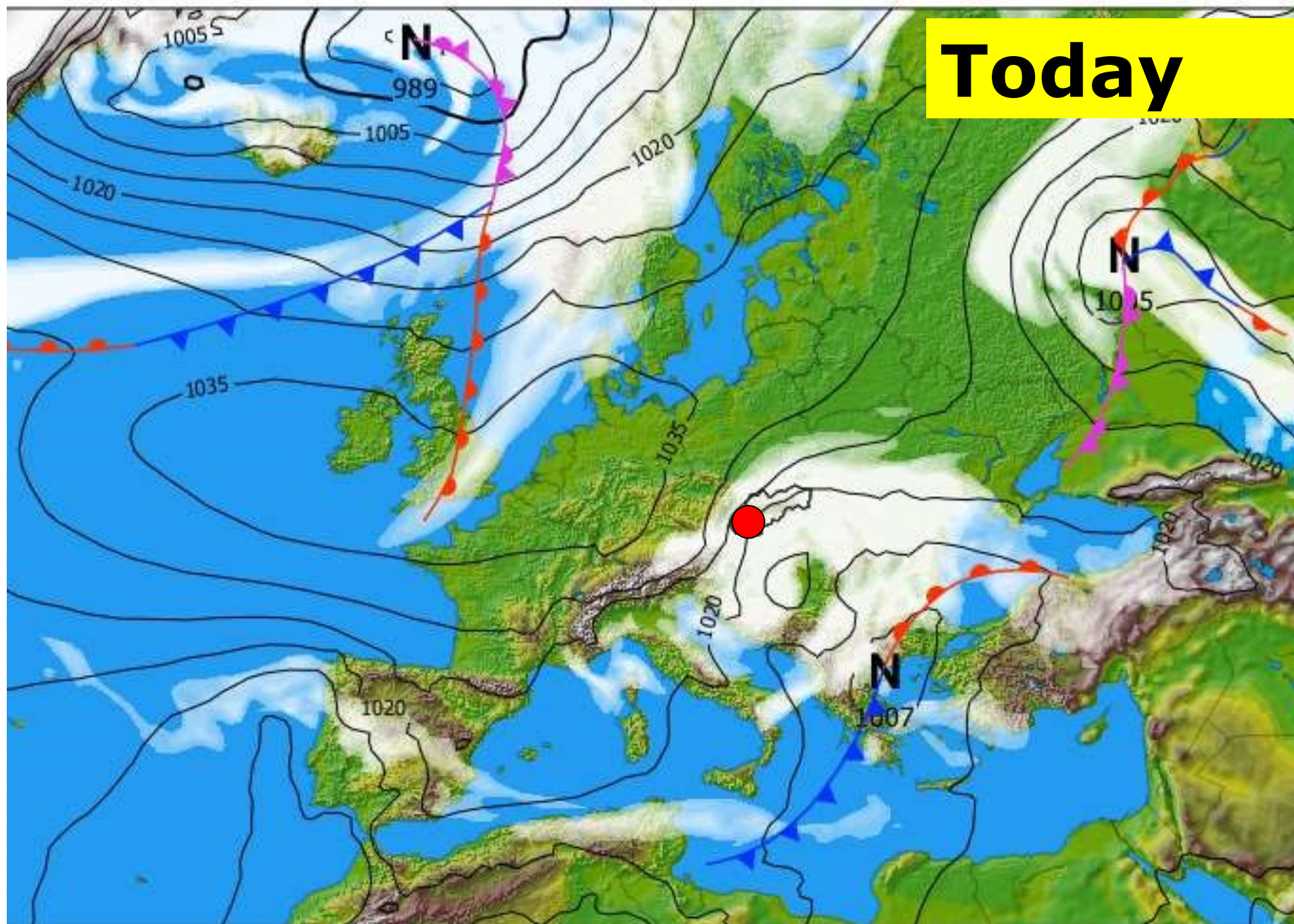
(c) SHMÚ - Prízemné tlakové pole - štvrtok 20.04.2017 00:00 UTC
